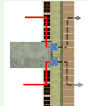
Fachada autoportante STRUCTURA-GHAS: R_A: 55,2 dBA R_{Atr}: 50 dBA R_w (C; C_{tr}) = 56 (-2; -6) dB
