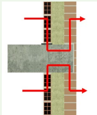
Fachada confinada convencional: R_A: 50 dBA R_{Atr}: 47 dBA R_w (C; C_{tr}) = 50 (0; -3) dB
